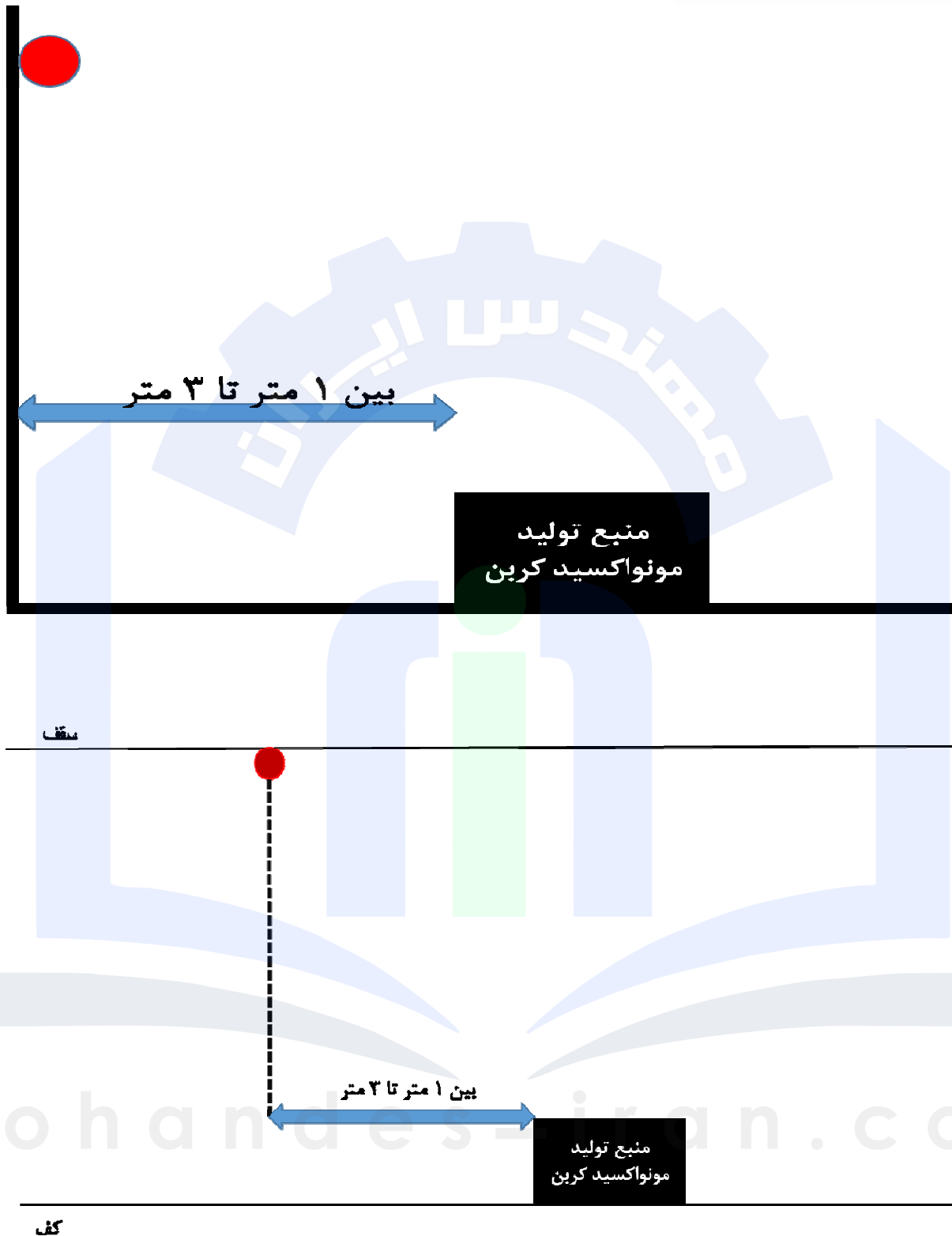
شکل (۳): فاصله آشکارساز نصب شده از منبع بالقوه تولید مونواکسید کربن
