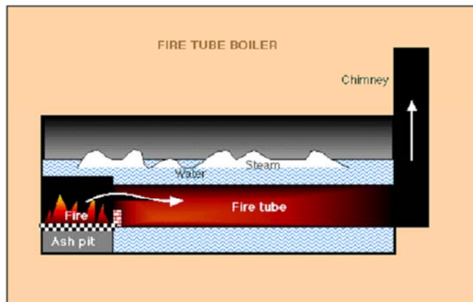
شکل 13-3- نمونه يك جوش آور فایر تیوب
